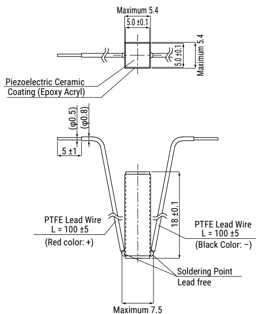
AE0505D18H18DF
