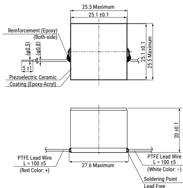
AE2525D15DF
