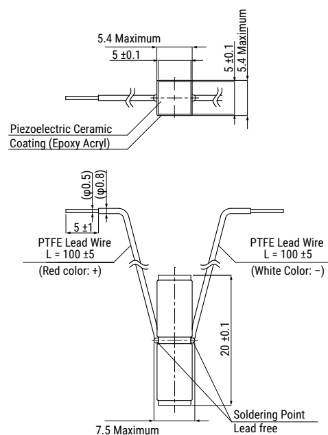
AE0505D16DF
